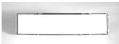
Ersatzabdeckung für Namensschildtaster Modell 630 +650 mit glatter Taste Aussenmaß 57,1mm x 14,4mm Schriftfeld 53,8 x 12mm *lieferbar solange Vorrat reicht
